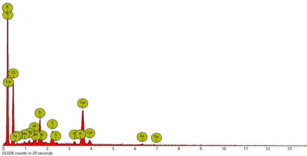
Bild 2: EDX-Spektrum zur Übersichtsaufnahme
