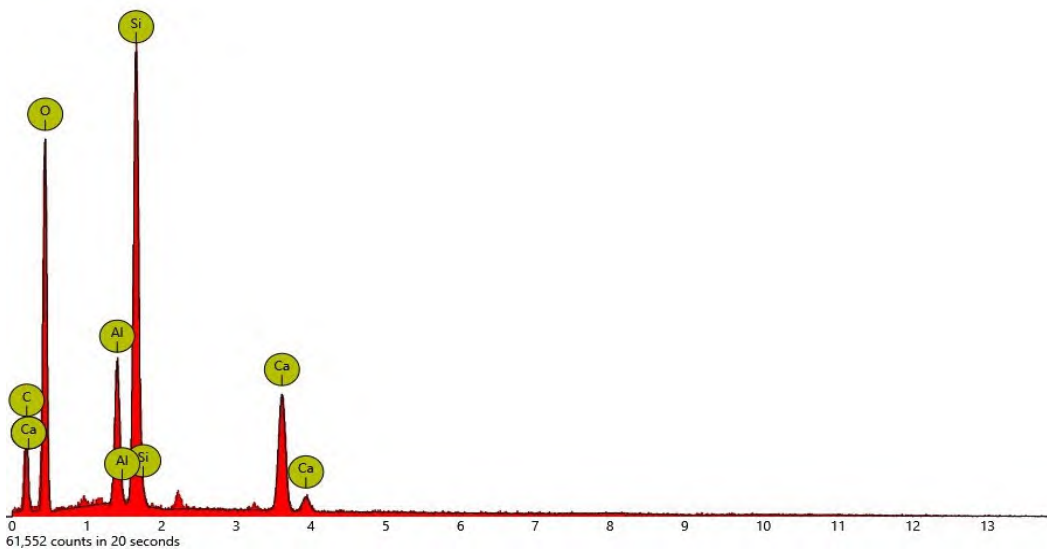
Bild 4: EDX-Spektrum Aluminiumsilikatwolle
